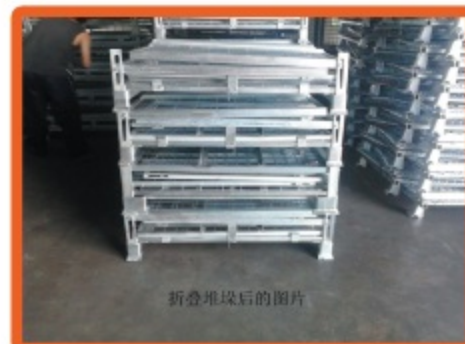
collapsible 瓶胚笼折叠效果
